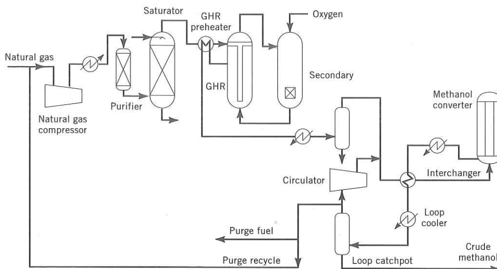
Fig. 4. ICI LCM process.
